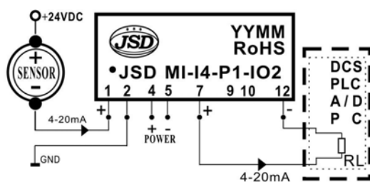
电流输入/电流输出 (I/I隔离)
