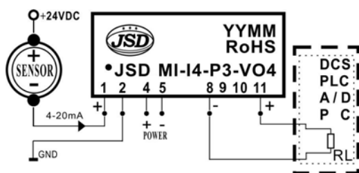
电流输入/电压输出 (I/V转换)
