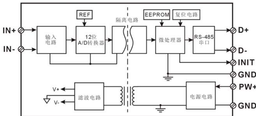
JSD AD11 模块内部框图
