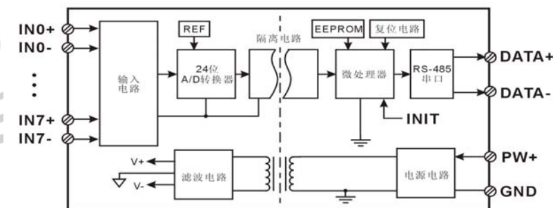
JSD81 内部方框图
