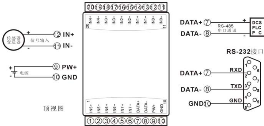
JSD81 转换器接线图
